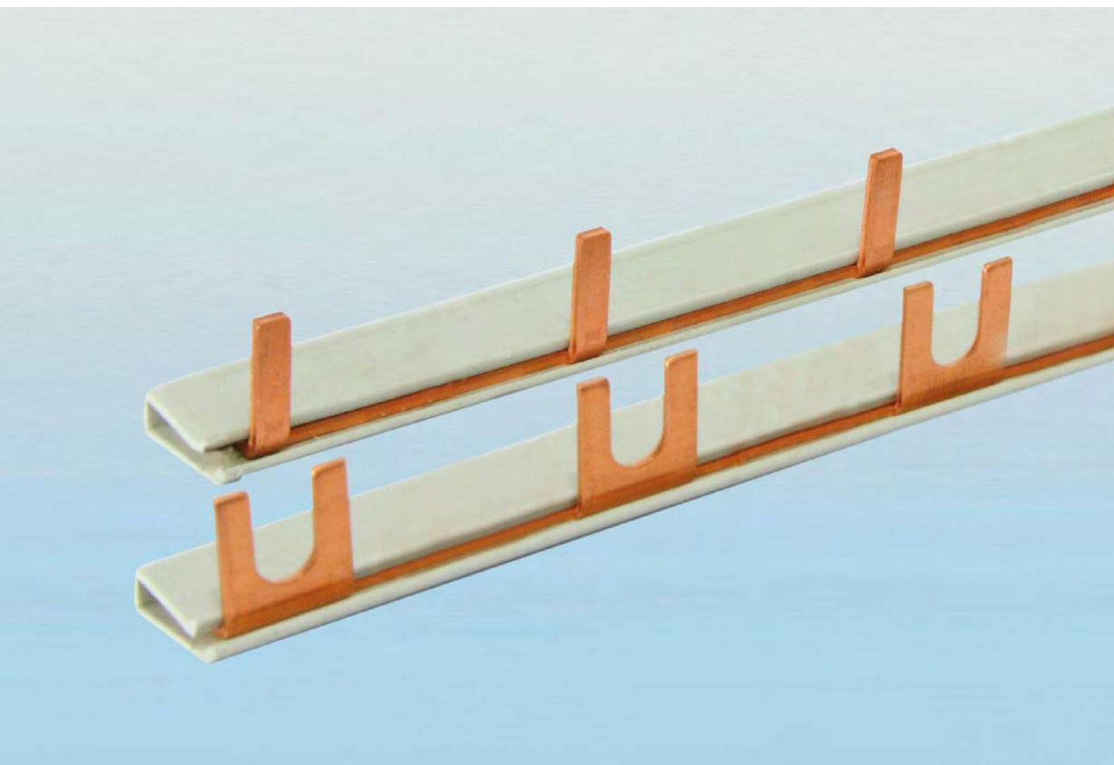
Phasenschiene für Hilsschalter H1 + H2 | Busbars for Auxiliary switch H1 + H2 | Peignes unipolaires pour Interrupteur auxiliaire H1 + H2
