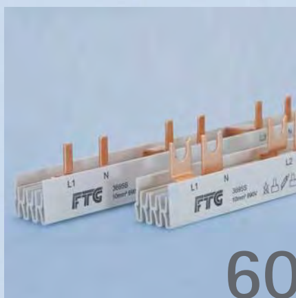
Phasenschienen für Hilfsschalter H1 + H2 Busbars for Auxiliary switch H1 + H2 Peignes unipolaires pour Interrupteur auxiliaire H1 + H2
